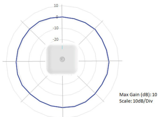
8x8 5 GHz Azimuth
