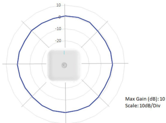
4x4 2.4 GHz Azimuth
