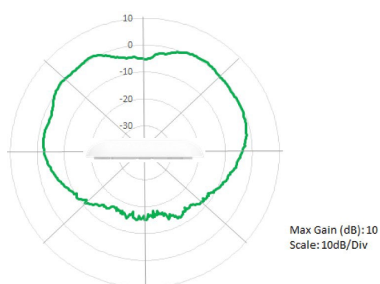
8x8 5 GHz Elevation
